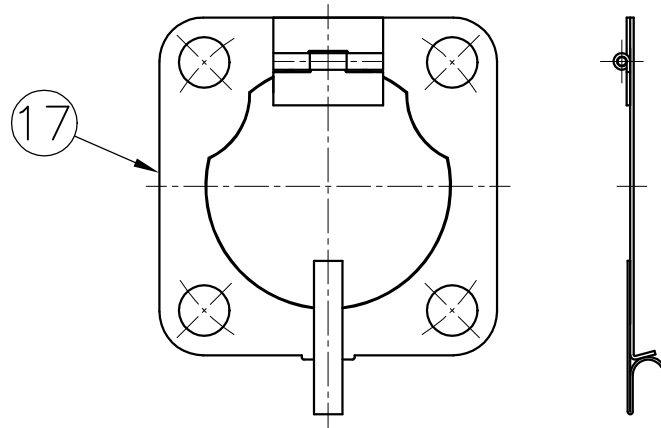
保護カバー詳細
