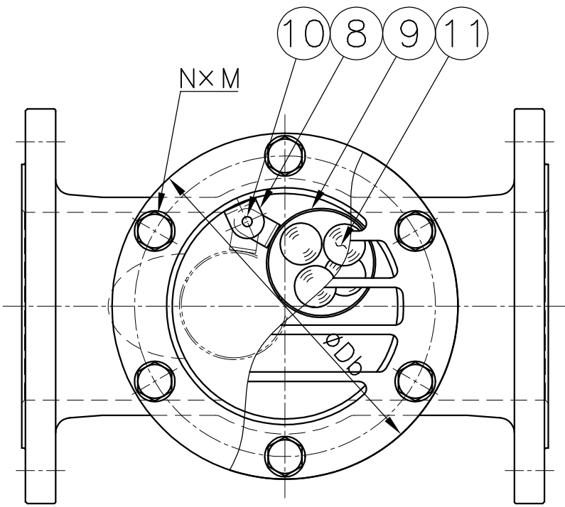
矢視 X-X
