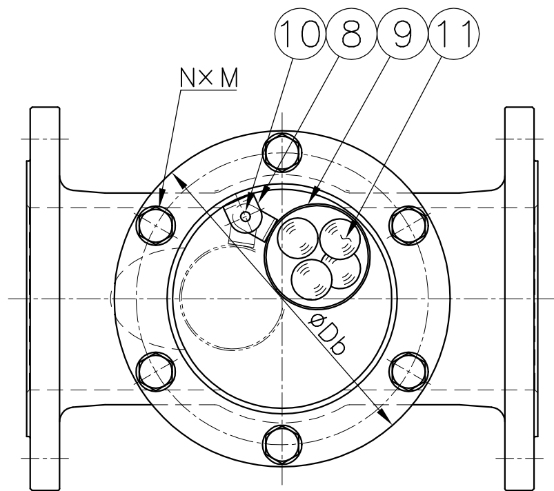
矢視 X-X
