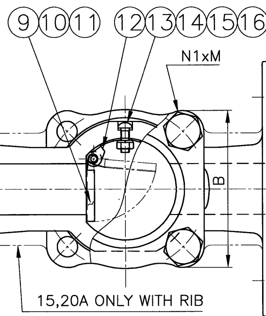
矢視 X-X
