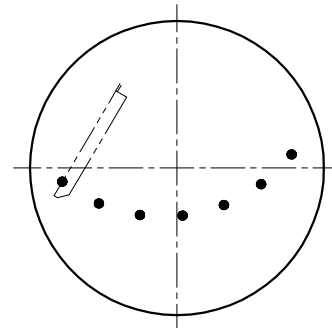
目盛詳細 (65-150A)
