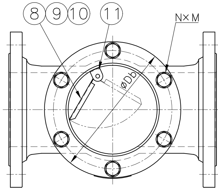
矢視 X-X
